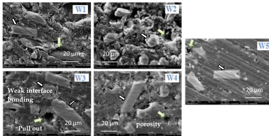
Fig-5: SEM-SE images of composites
